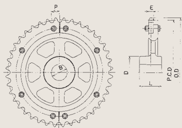
組合せ形
