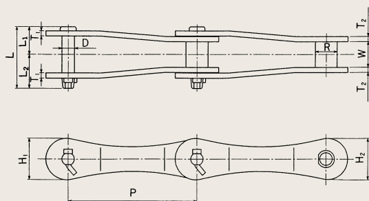
OSV形ステンレスチェーン
