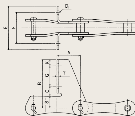
SF4アタッチメント
